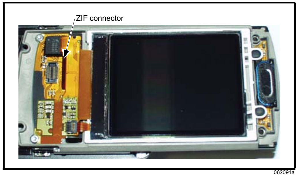
Figure 27. Unlocking the Display Module ZIF Connector
