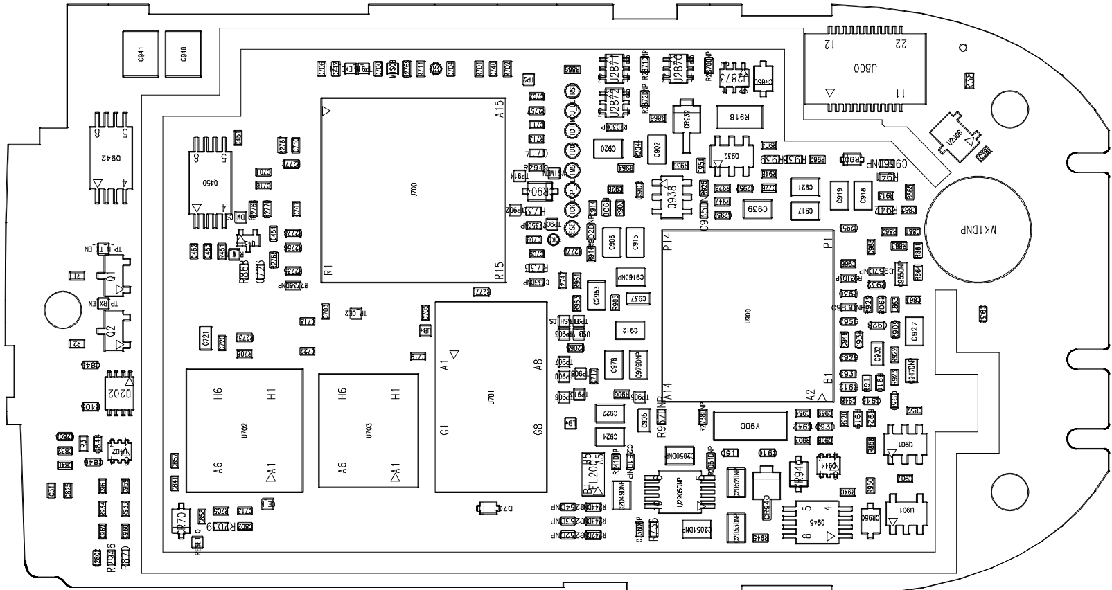
LAYER 1 ASSEMBLY
